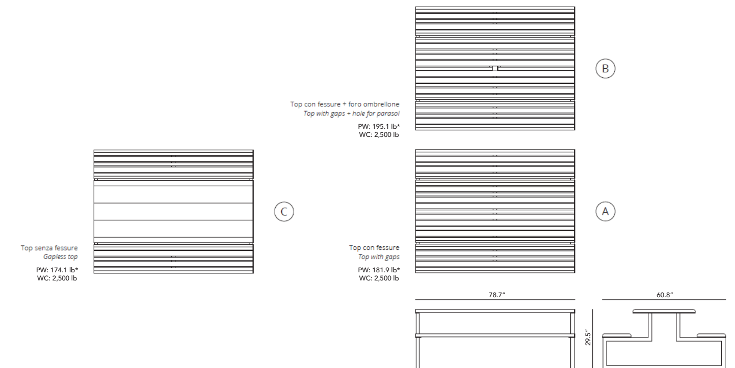
Tavolo picnic / Picnic table
