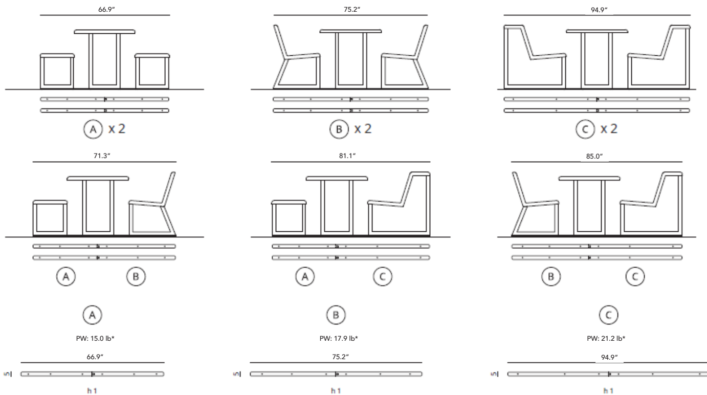
Barre di unione / Linking plates
