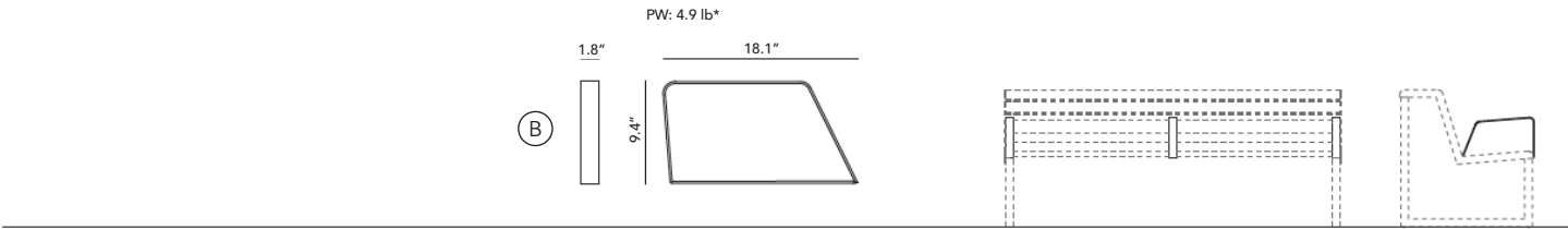
Bracciolo panche con schienale / Armrest benches with backrest
